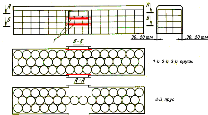
Рисунок 27 - Размещение и крепление рулонов бумаги диаметром 850 мм, шириной 594 мм: 1 – доска ограждения
