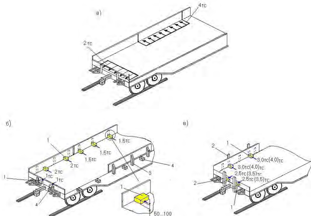
Рисунок 38- Схемы нагружения бортов платформ 1 – упорный брусок; 2 – короткая стойка из дерева или металла; 3 – клиновой запор; 4 –стойчатая скоба
