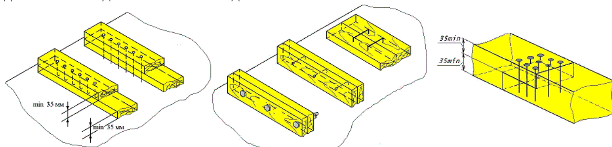
Рисунок 15 – Способы изготовления составных подкладок, прокладок
