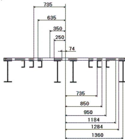
Рисунок 3 – Зоны передачи нагрузок на настил пола платформы
