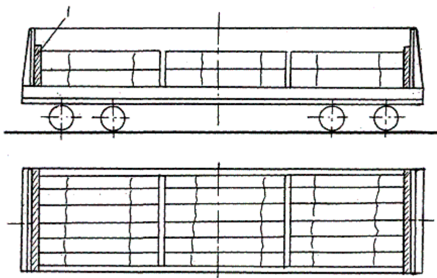
Рисунок 16 1 – торцовый щит
