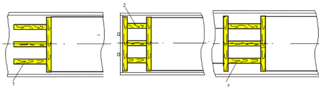
Рисунок 9 – Установка распорных и упорных брусков и рам для крепления грузов в вагонах от поступательных смещений 1 – брусок упорный; 2 – брусок распорный
