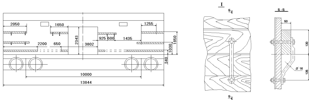
Рисунок 2 - Расположение деталей несъемного оборудования внутри кузова вагона:
