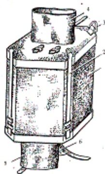
Рисунок 64 – Специализированный контейнер МК – Л 1 – корпус; 2 – грузовая лента; 3 – серьга; 4 – загрузочный рукав; 5 – разгрузочный рукав; 6 – клапан
