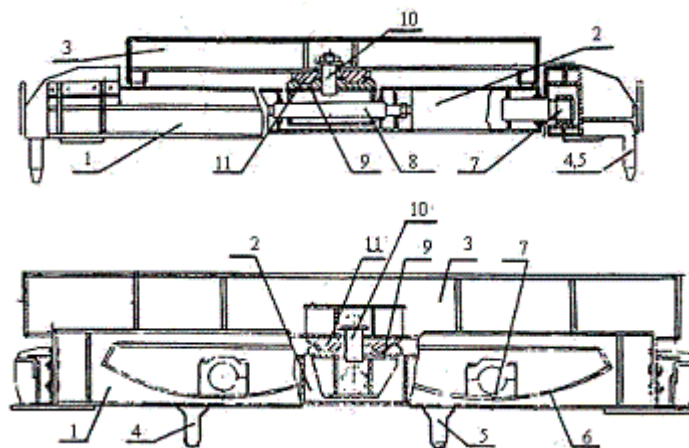
Рисунок 53 Турникетная опора типа Гипростроймост
