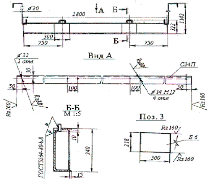
Рисунок 41 – многооборотный упор для специализированных контейнеров СК-2-3,2
