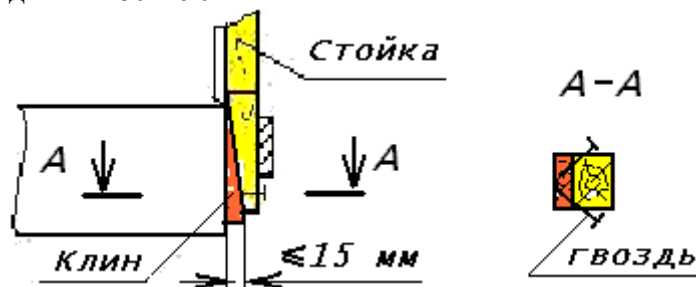
Рисунок 17 – Крепление стойки в стоечной скобе платформы
