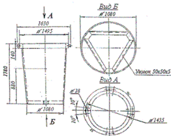
Рисунок 48 – Спецконтейнер Гипроцветмета
