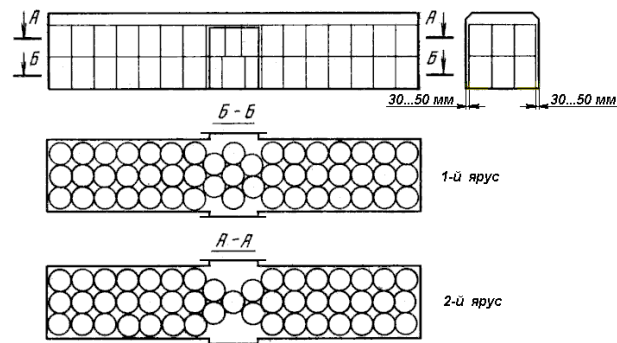
Рисунок 20 – Размещение и крепление рулонов бумаги диаметром 800 мм, шириной 940-1400 мм
