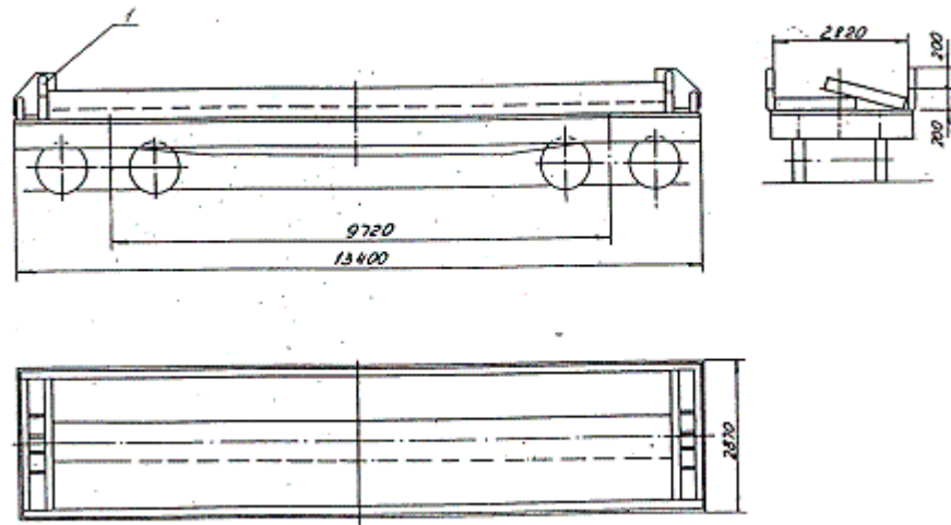
Рисунок 104 1 – балка упорная
