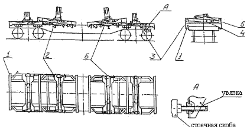
Рисунок 30-Размещение и крепление порожних турникетов для железобетонных вибрированных стоек на одной платформе
