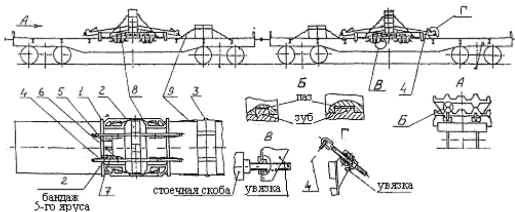
Рисунок 29-Размещение и крепление порожнего турникета для ж.б. центрифугированных стоек на сцепе двух платформ
