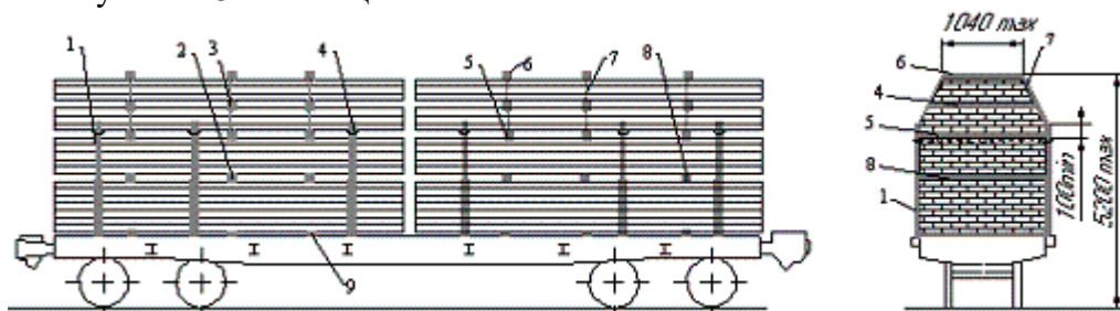
Рисунок 33 – Непакетированные пиломатериалы на платформе 1 – стойка; 2 – прокладка; 3 – прокладка «шапки»; 4 – скрепление стоек; 5 – удлиненная прокладка; 6 – верхний поперечный брусок; 7 – увязка «шапки»; 8 – утолщенная прокладка; 9 – подкладка
