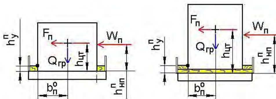
Рисунок 32-Варианты расположения упоров от опрокидывания груза в поперечном направлении
