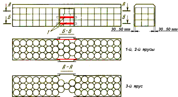
Рисунок 21 – Размещение и крепление рулонов бумаги диаметром 800 мм, шириной 710-930 мм: 1 – доска ограждения
