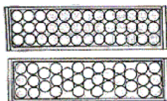
Рисунок 69 – Размещение в полувагоне контейнеров МКР-М и МКР-С
