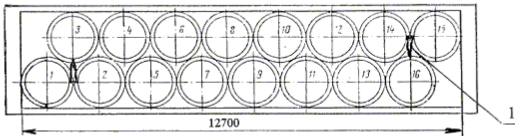
Рисунок 44 – Размещение контейнеров в полувагоне объемом кузова от 76 до 83 м 3 1 – увязка
