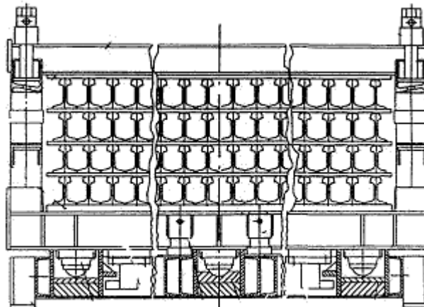
Рисунок 33-Железнодорожные рельсы на турникете
