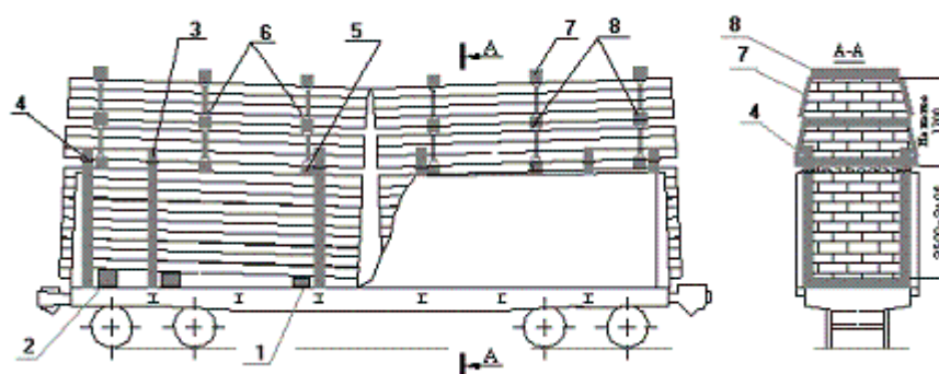
Рисунок 34 – Непакетированные пиломатериалы в полувагоне 1 – подкладка; 2 – утолщенная подкладка; 3 – стойка; 4 – скрепление стоек; 5 – удлиненная прокладка; 6 – прокладка «шапки»; 7 – верхний поперечный брусок; 8 – увязка «шапки»
