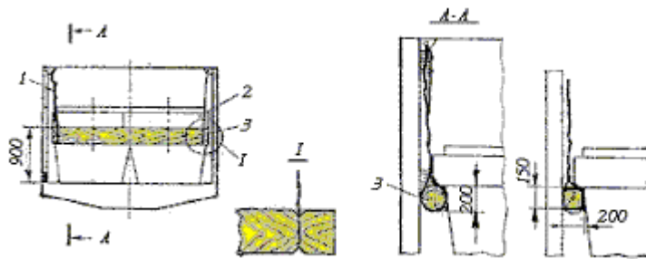
Рисунок 43 – установка упора из лесоматериалов 1 – подвеска; 2 – контейнер; 3 – упор
