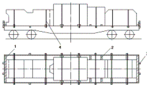
Рисунок 16 1 – брусок упорный; 2 – брусок распорный; 3 – стойка короткая; 4 – обвязка
