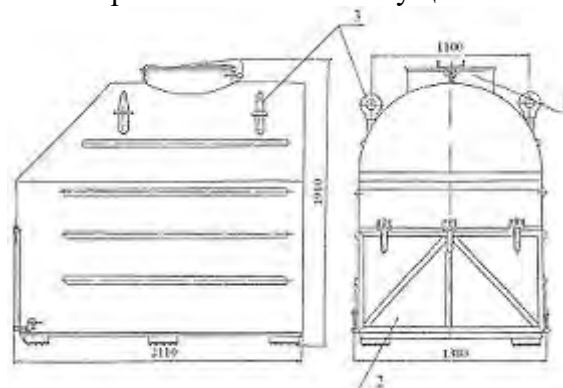
Рисунок 27 – спецконтейнер КИУ – 5М
