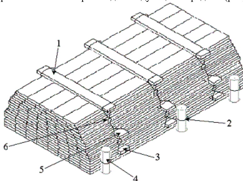
Рисунок 35 Формирование «шапки» непакетированных пиломатериалов 1 – поперечный брусок; 2 – верхнее скрепление стоек, 3 – удлиненная прокладка; 4 – стойка; 5 – прокладка; 6 – увязка
