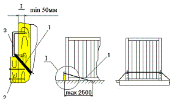
Рисунок 12 – Установка наклонных обвязок для крепления деревянных ящиков: 1-обвязка; 2 – брусок; 3 – скоба строительная
