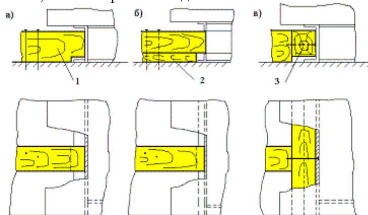
Рисунок 10 - Установка упорных брусков: а) – с подрезом бруска , б) - на подкладке), в) - с промежуточным упорным бруском 1 – брус упорный; 2 – доска подкладная, 3 – брус упорный промежуточный
