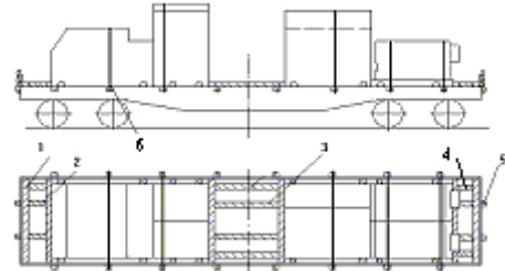
Рисунок 17 1 – брусок упорный; 2,3,4 – брусок распорный; 5 – стойка короткая; 6 – обвязка
