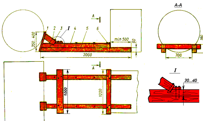
Рисунок 19 - Конструкция распорной рамы:
