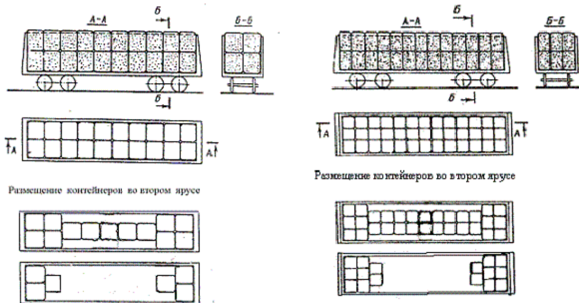
Рисунок 65 Размещение контейнеров в два ряда по ширине полувагона
