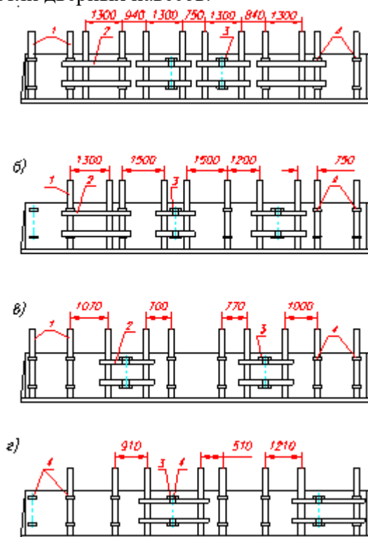
Рисунок 1 – Установка стоек в полувагоне при количестве штабелей 4 и более
