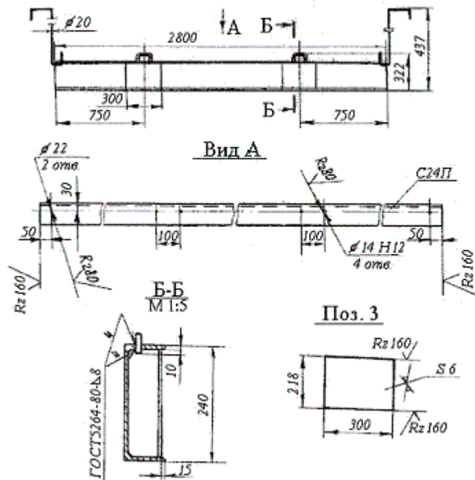
Рисунок 42 - многооборотный упор для специализированных контейнеров СК 2 – 5
