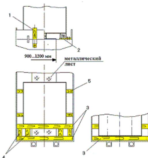
Рисунок 13 – Установка груза у торцового борта платформы 1 – стойка; 2 – подкладка выравнивающая; 3 – упорный брусок; 4, 5 – распорные бруски
