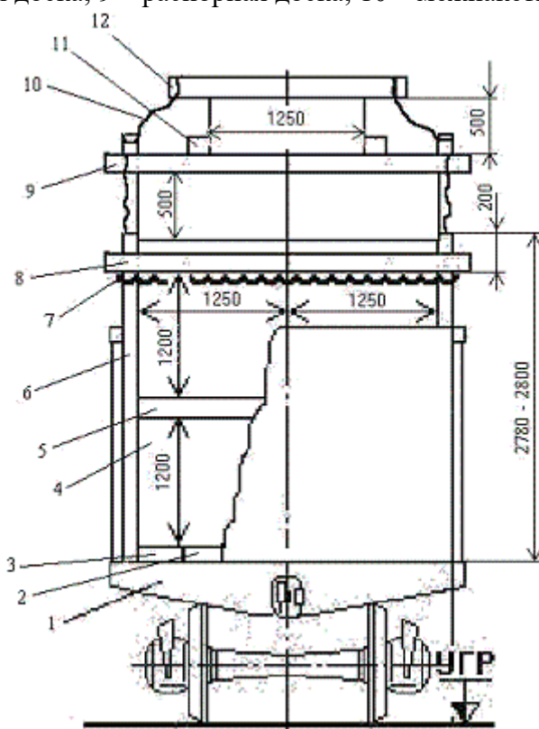
Рисунок 54 – формирование «шапки» по варианту 3 в полувагоне 1 – полувагон; 2 – торцовый упор; 3 – подкладка; 4 – пакет прямоугольной части штабеля; 5 – прокладка; 6 – стойка; 7 – крепление стоек; 8 – удлиненная прокладка; 9 – промежуточная удлиненная прокладка; 10 – увязка; 11 – упорная доска; 12 – прижимной брусок
