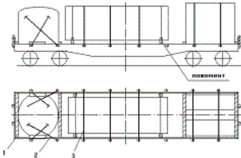
Рисунок 16 1 – брусок упорный; 2 – брусок распорный; 3 – стойка короткая; 4 – обвязка
