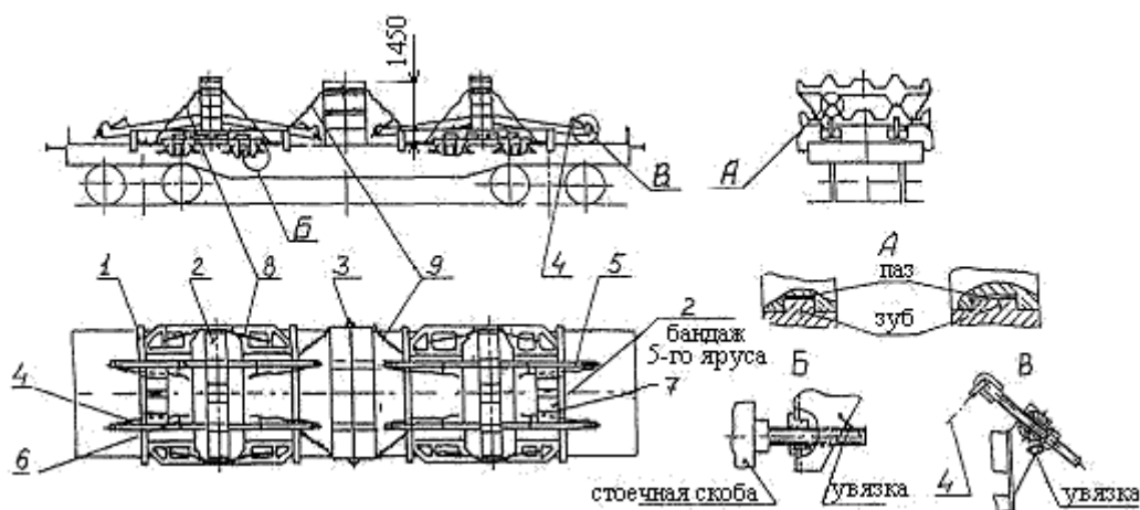
Рисунок 28 - Размещение и крепление порожнего турникета для ж.б. центрифугированных стоек на одной платформе
