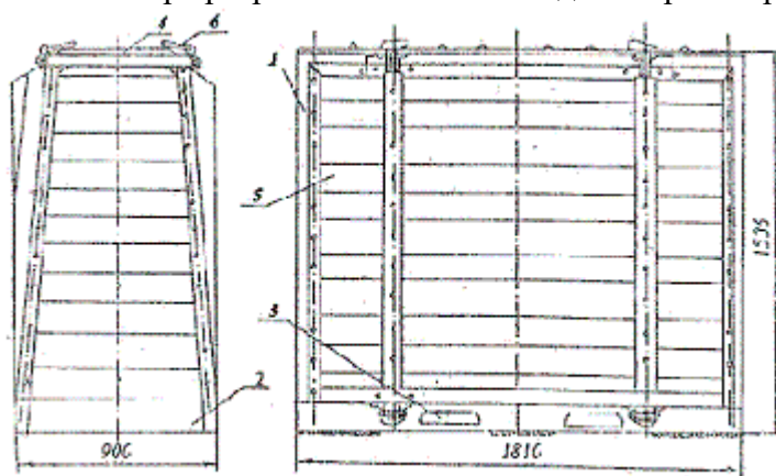
Рисунок 53 – спецконтейнер ПКС - 2,85
