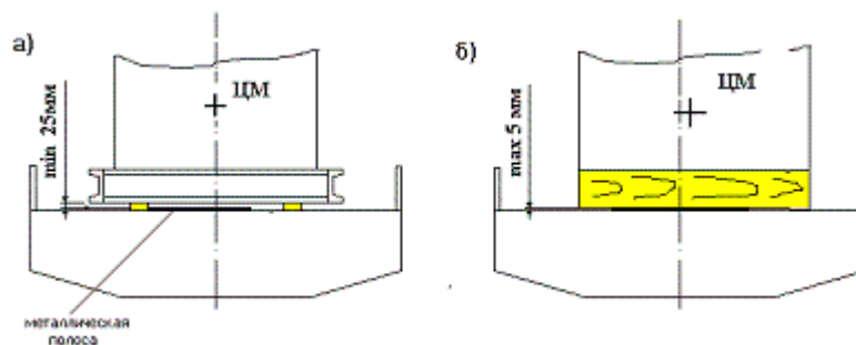
Рисунок 4- Установка груза на дерево-металлический пол: а) на двух подкладках; б) без подкладки
