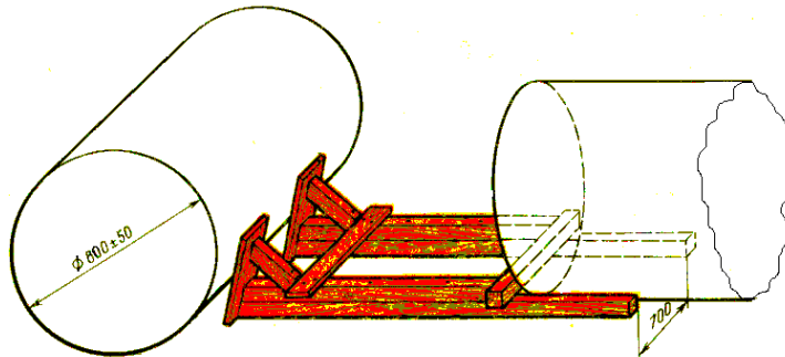
Рисунок 18 - Установка распорной рамы
