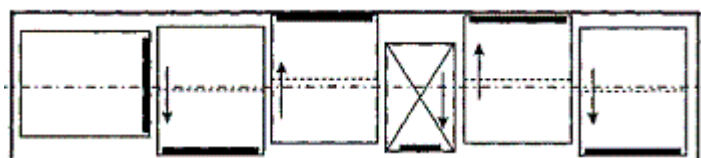
Рисунок 5 – Размещение в полувагоне с внутренней длиной кузова 12700 мм разнотипных контейнеров; количество контейнеров УУК-3, УУК-3(5) – нечетное
