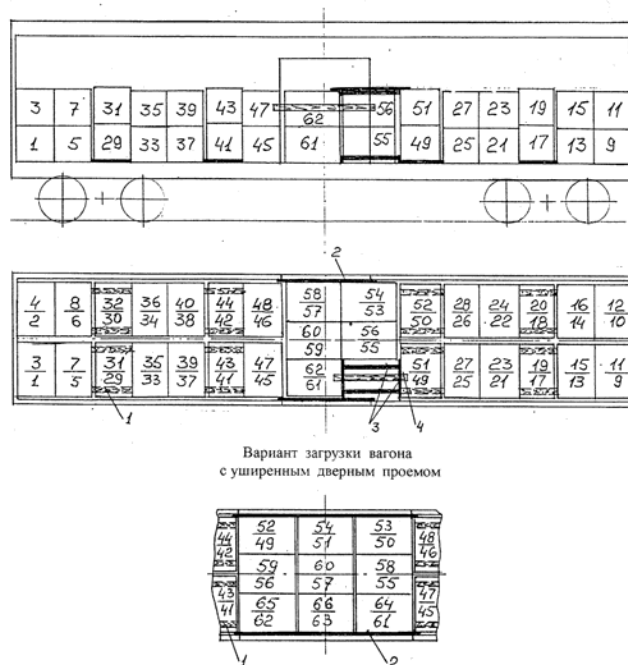
Рисунок 15 – Размещение и крепление транспортных пакетов с керамической плиткой:
