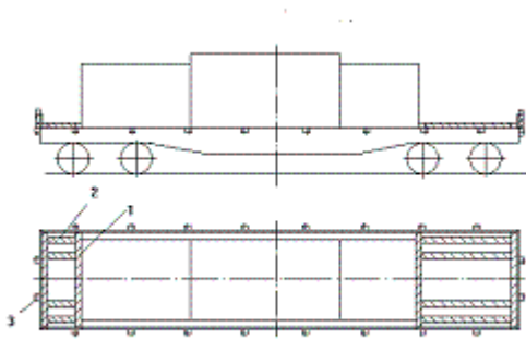
Рисунок 14 1,2 – брусок упорный
