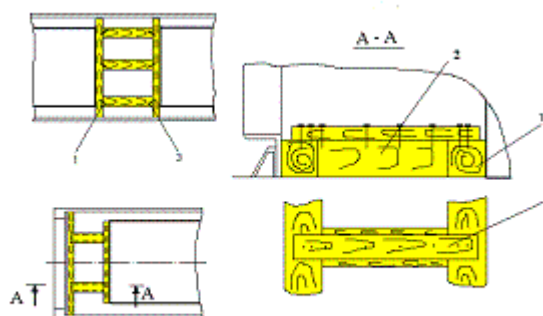
Рисунок 8 – Установка упорных и распорных рам в полувагоне: 1 – упорный брусок; 2 – распорный брусок; 3 – скоба строительная; 4 – доска накладная
