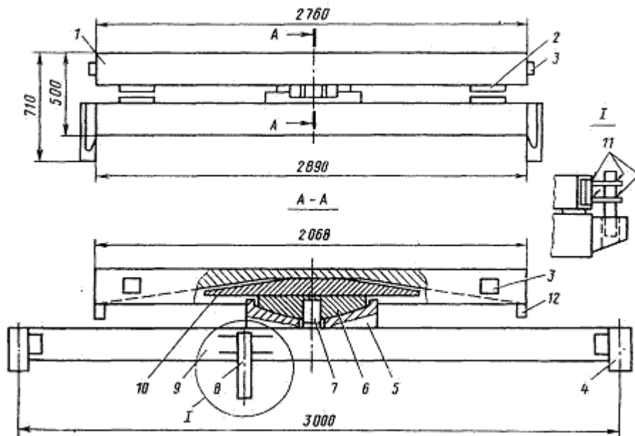
Рисунок 35 Турникетная опора типа ЦНИИ МПС
