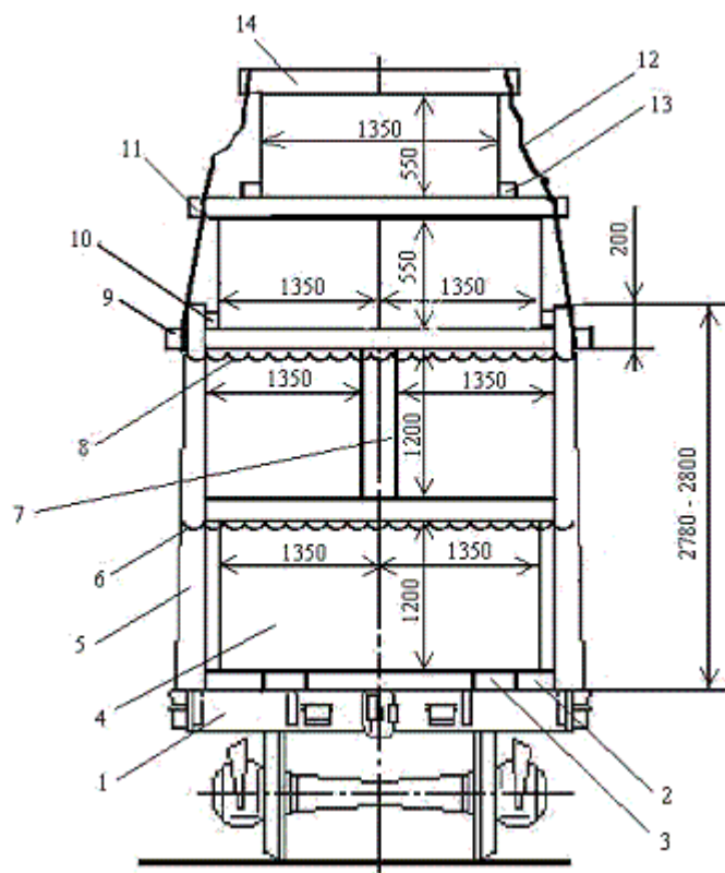
Рисунок 55 – формирование «шапки» по варианту 3 на платформе 1 – платформа; 2 – подкладка; 3 – торцовый упор; 4– пакет прямоугольной части штабеля; 5 – прокладка; 6 – среднее скрепление стоек; 7 – межпакетное заполнение; 8 – верхнее скрепление стоек; 9 – удлиненная прокладка; 10 – распорная доска; 11 – промежуточная удлиненная прокладка; 12 – увязка; 13 – упорная доска; 14 – прижимной брус
