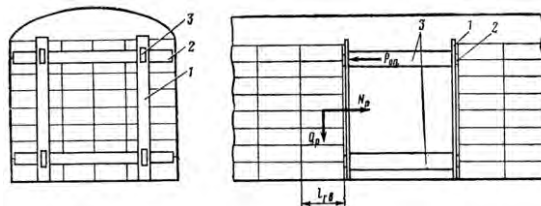
Рисунок 6 – Установка распорной конструкции в междверном пространстве вагона
