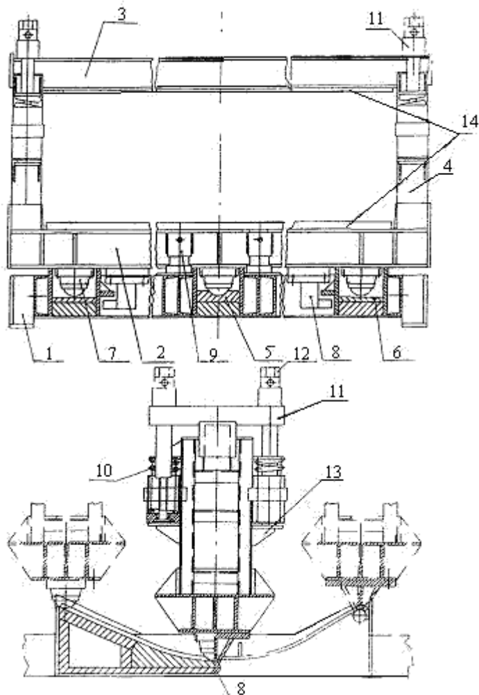
Рисунок 31-Турникетная опора типа УО ВНИИЖТ.
