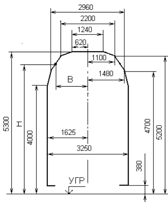
Рисунок 3 – Очертание зонального габарита погрузки
