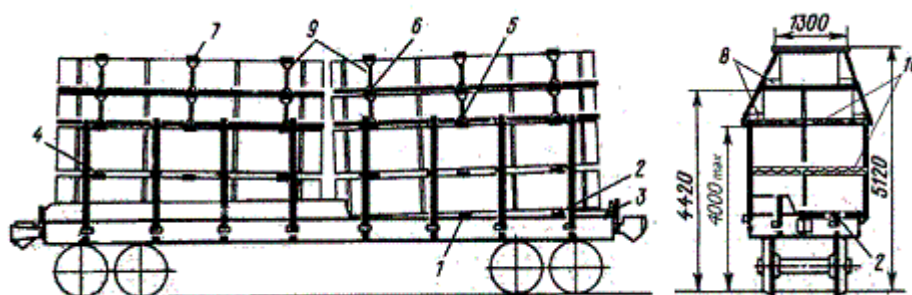
Рисунок 48 – Размещение пакетов пиломатериалов на платформе
