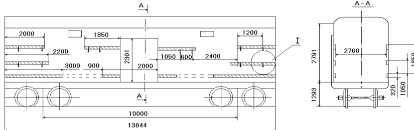
Рисунок 1 - Кузов вагона
