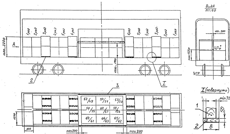
Рисунок 14 – Размещение и крепление транспортных пакетов огнеупорных изделий с уширенным дверным проемом
