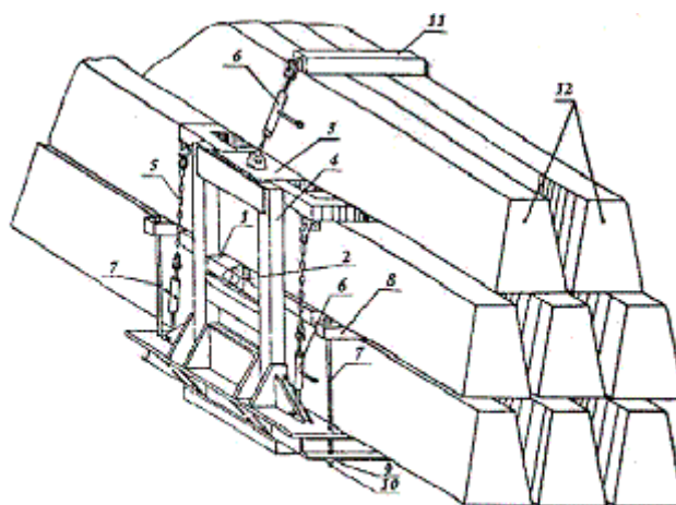
1-балка второго яруса; 2-груз; 3-балка третьего яруса; 4-стойка; 5-цепь; 6-винтовой механизм; 7-шпилька; 8-балка; 9-рейка; 10-контргайка; 11-короткая балка; 12-контейнер
