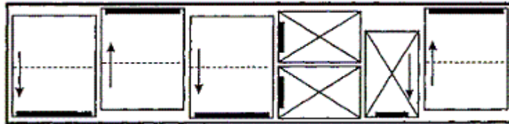
Рисунок 8 – Размещение контейнеров в контейнеровозах с обшивкой стен, имеющих четыре специальных отверстия в боковых стенах кузова вагона. Количество контейнеров УУК-3, УУК-3(5) – нечетное.
