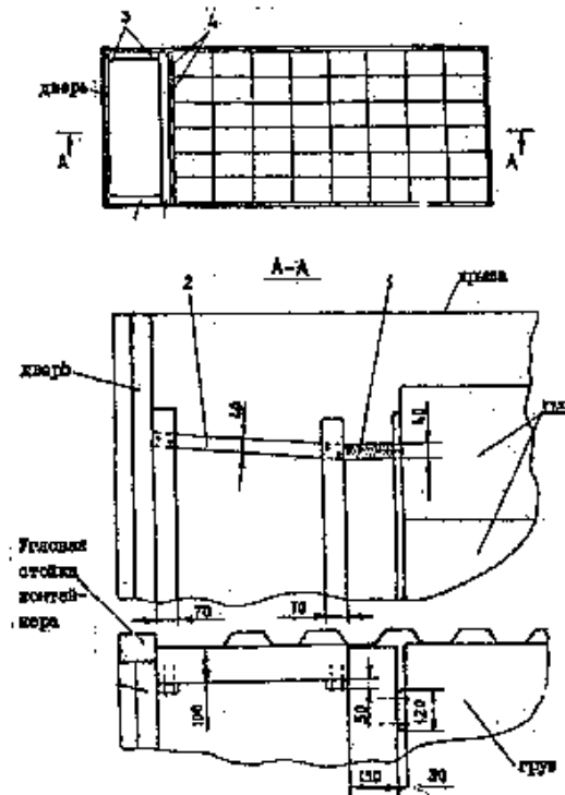
Рисунок 1 (Вид сверху контейнера).
