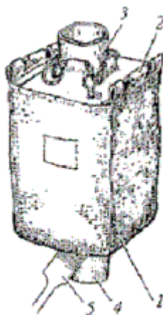
Рисунок 63 – Специализированный контейнер МК – П 1 – корпус; 2 – проушина; 3 – загрузочный рукав; 4 – разгрузочный рукав; 5 – клапан
