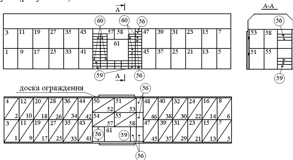
Рисунок 16 - Размещение транспортных пакетов, сформированных из мешков (номераами показан порядок загрузки транспортных пакетов. В кружках - с раскладкой отдельными мешками)
