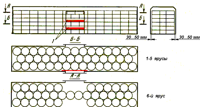
Рисунок 28 - Размещение и крепление рулонов бумаги диаметром 850 мм, шириной 420 мм:
