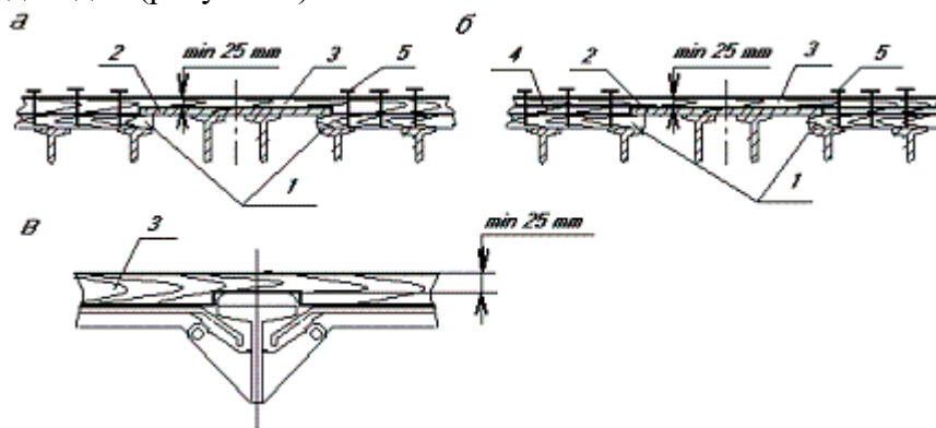
Рисунок 1 Устройство поперечных подкладок а, б – на платформах; в – в полувагоне.
