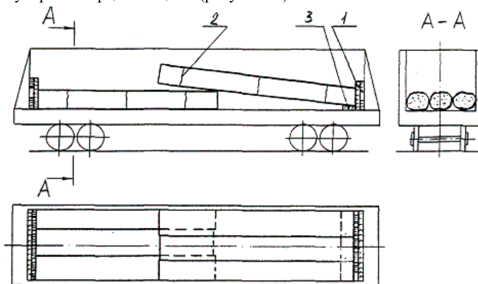
Рисунок 17 1 – торцовый щит; 2 – увязка; 3 – поперечная подкладка
