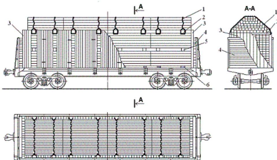
Рисунок 31 – Непропитанные шпалы в полувагоне
