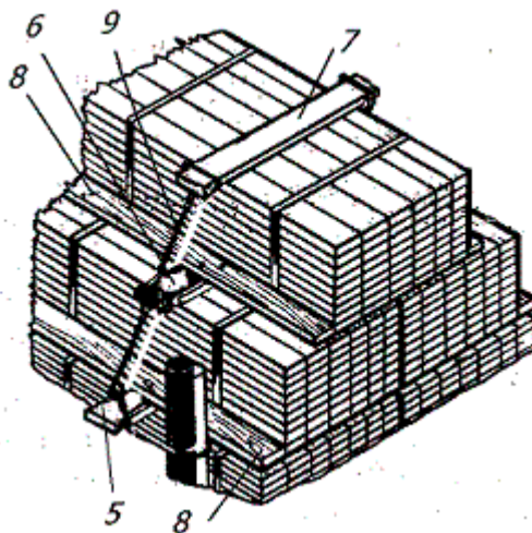
Рисунок 49 – формирование «шапки» из пакетов пиломатериалов 5, 6 – удлиненная прокладка; 7 – прижимной брусок; 8 – упорная доска; 9 – увязка «шапки»
