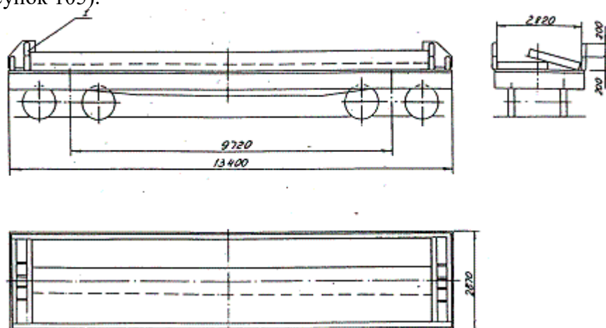
Рисунок 105 1 – балка упорная
