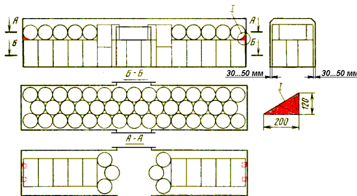
Рисунок 24 - Размещение и крепление рулонов бумаги диаметром 850 мм, шириной 1680 мм и 1260 мм
