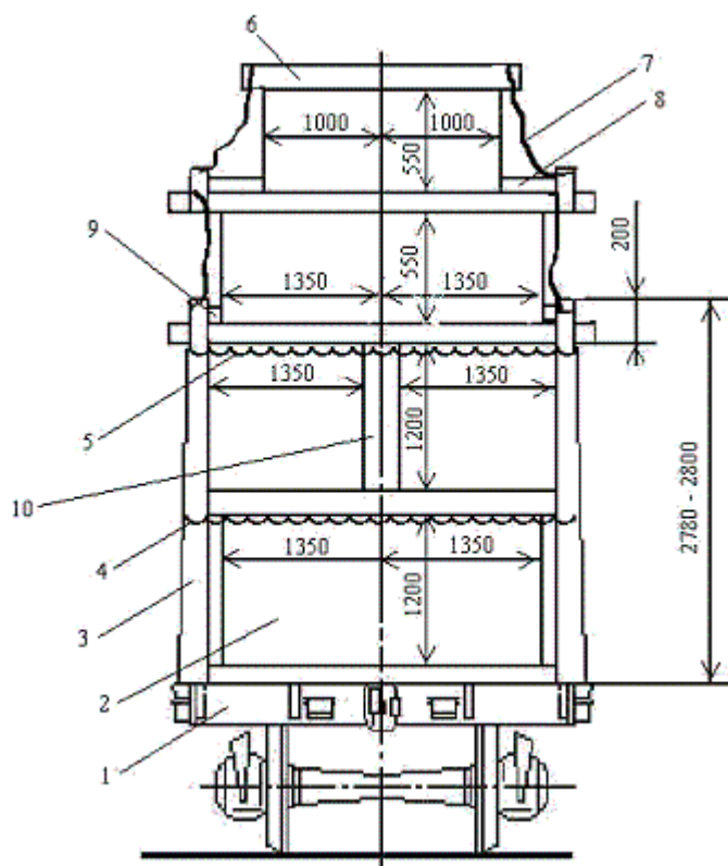
Рисунок 53 – формирование «шапки» по варианту 2 на платформе 1 – платформа; 2 – пакет прямоугольной части штабеля; 3 – стойка; 4 – среднее крепление стоек; 5 – верхнее крепление стоек; 6 – прижимной брусок; 7 – увязка; 8 – упорная доска; 9 – распорная доска; 10 – межпакетное заполнение
