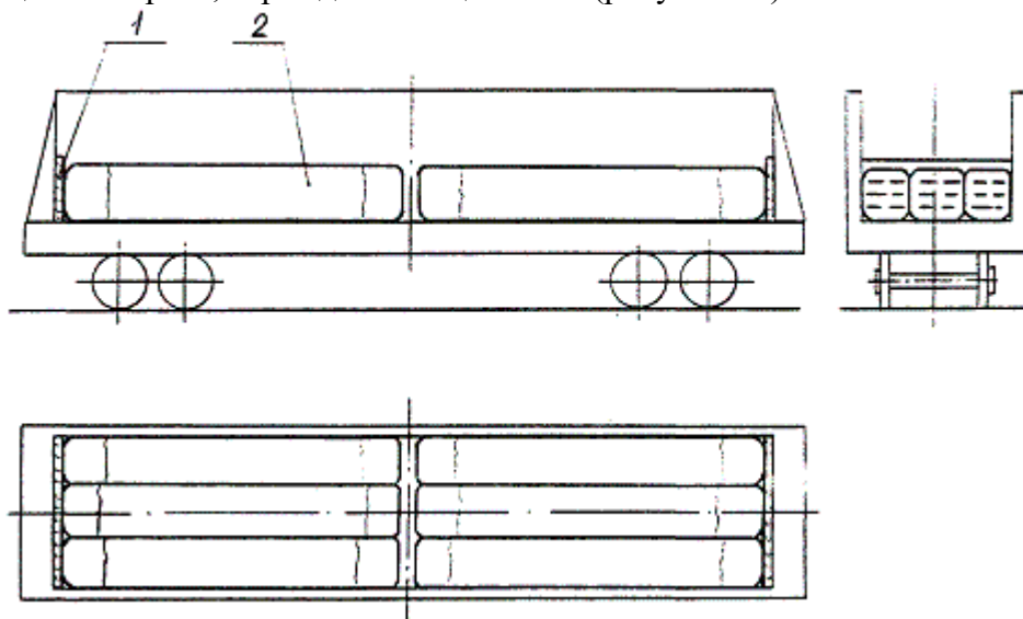
Рисунок 10 1 – торцовый щит; 2 – связка
