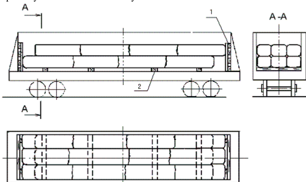
Рисунок 11 1 – торцовый щит; 2 – поперечная подкладка
