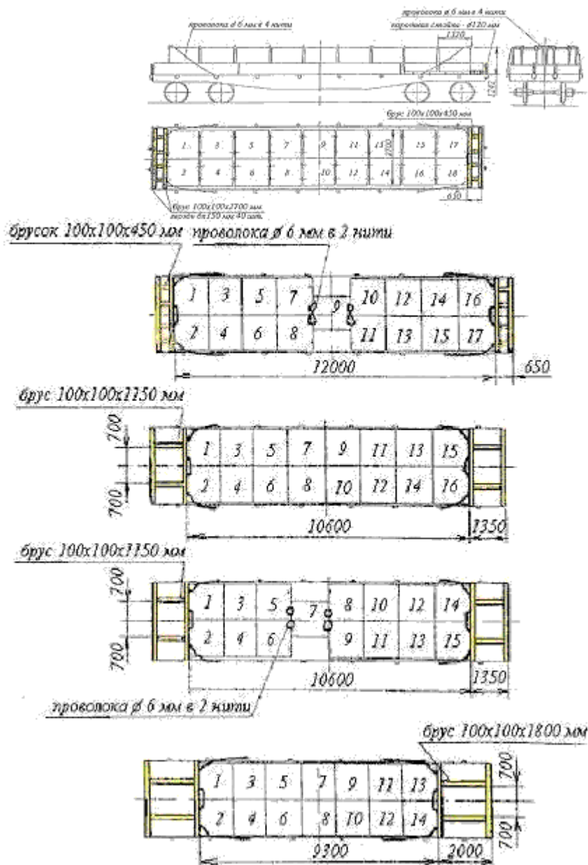
Рисунок 50 – Схемы размещения и крепления контейнеров
