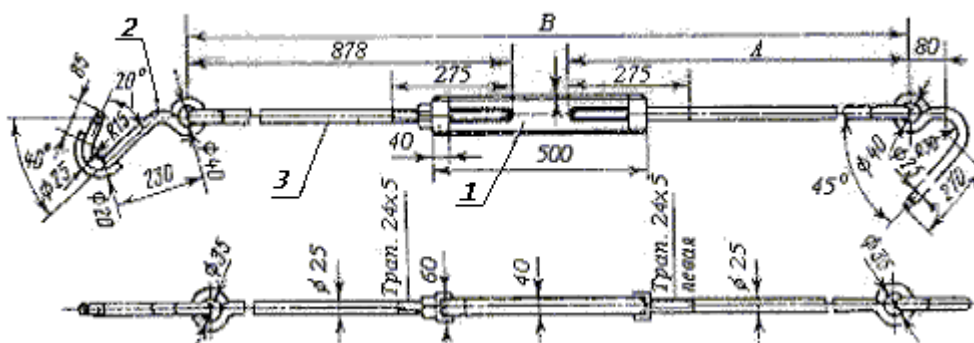
Рисунок 37 – инвентарная растяжка
