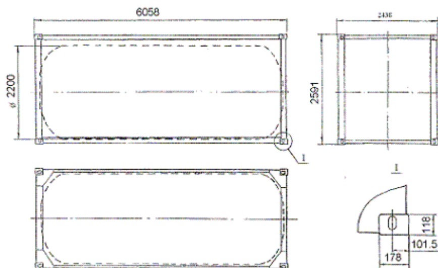
Рисунок 56 – Спецконтейнер-цистерна типа 1M01 (или 1M05)
