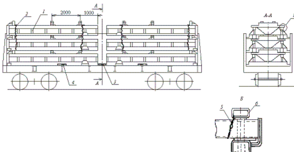
Рисунок 140 – Схема погрузки рам черт. 64295-1.1СБ АО «Северсталь» при возврате 1- рама в сборе с поперечной балкой; 2- обвязка; 3- центральная распорная клетка (либо пакет брусков); 4- боковая распорная клетка; 5- увязка; 6- штырь фиксатор
