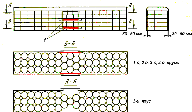
Рисунок 22 – Размещение и крепление рулонов бумаги диаметром 800 мм, шириной 485-550 мм: 1 – доска ограждения
