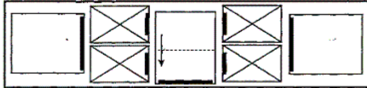
Рисунок 7 – Размещение разнотипных контейнеров в контейнеровозах без обшивки стен, с торцевым ограждением в виде упорной балки, закрепленной с внутренней стороны угловых стоек, а также в контейнеровозах с обшивкой стен, имеющих в боковых стенах кузова специальные отверстия. Количество контейнеров УУК-3, УУК-3(5) – четное.
