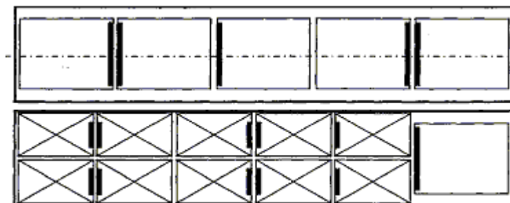
Рисунок 1 – Размещение контейнеров на универсальной платформе с внутренней длиной 13300 мм
