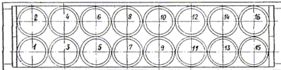
Рисунок 45 – Размещение контейнеров в полувагоне объемом кузова 85 м 3
