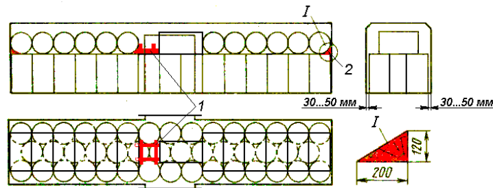
Рисунок 23 – Размещение и крепление рулонов бумаги диаметром 850 мм, шириной 1680 мм:
