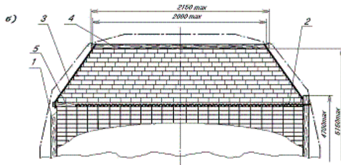
Рисунок 36 – Максимальные допускаемые размеры «шапки»: а) – в основном габарите погрузки; б) – в зональном габарите 1 – стойка; 2 – верхнее скрепление стоек; 3 – увязка шапки; 4 – поперечный брусок; 5 – удлиненная прокладка; 6 – прокладка шапки
