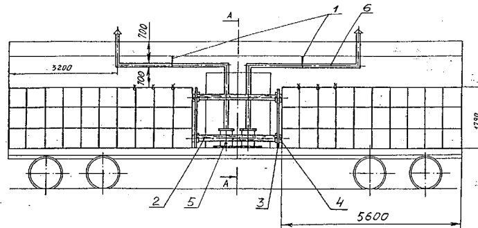
Рисунок 4 – Размещение тарных штучных грузов в вагоне с сопровождением проводниками
