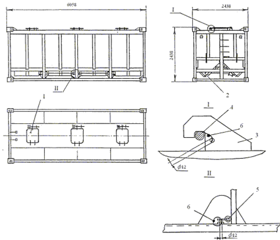
Рисунок 29 – спецконтейнер КРЦ – 2
