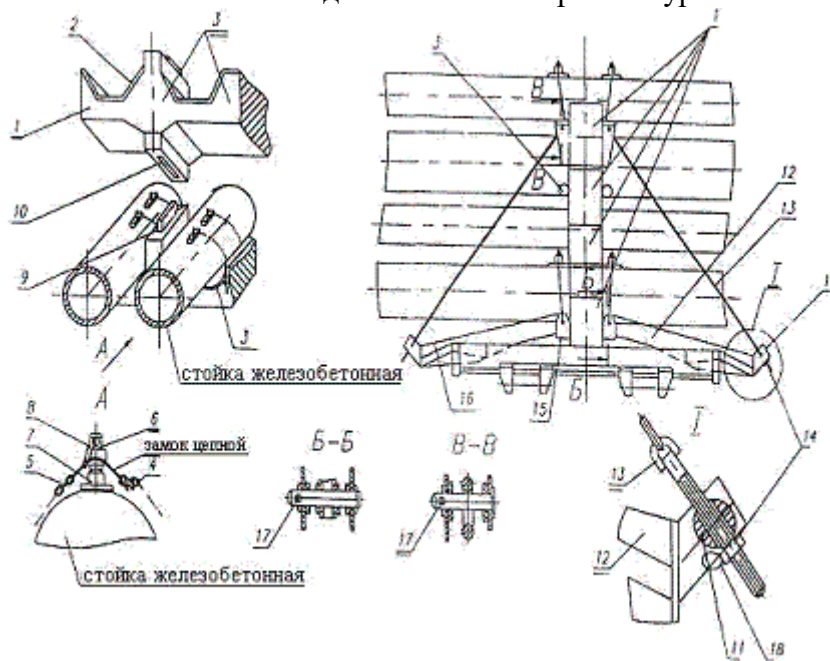
Рисунок 18- Комплект крепления для ж.б. центрифугированных стоек
