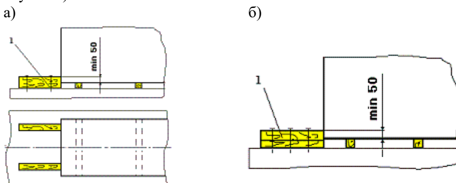
Рисунок 7 – Установка упорных брусков: а – монолитных; б – составных: по высоте 1 – упорный брусок
