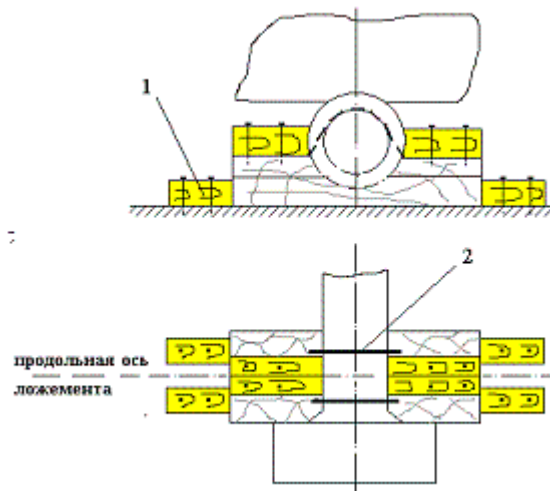
Рисунок 11 – Рекомендуемое крепление груза на ложементе упорными брусками 1 – брус упорный; 2 - обвязка
