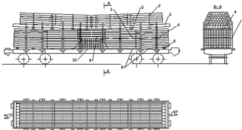
Рисунок 30 – Непропитанные шпалы на платформе
