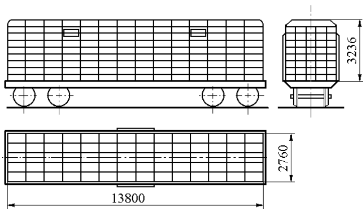
Рисунок 8. Размещение и крепление тюков соломы
