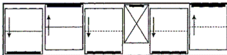
Рисунок 2 – Размещение контейнеров в полувагоне с внутренней длиной кузова 12056...12228 мм
