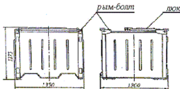
Рисунок 18 – спецконтейнер СК-1-3,4
