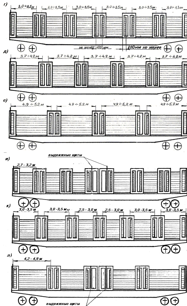
Рисунок 74 – Размещение круглых лесоматериалов и пиломатериалов длиной от 2,0 до 5,2 м
