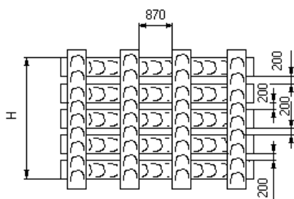
Рисунок 3. Деревянный щит ограждения
