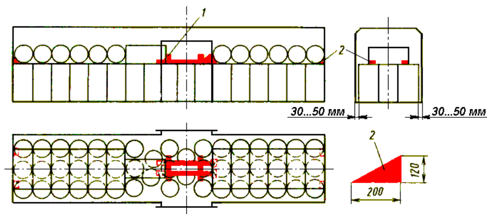
Рисунок 17 - Размещение и крепление рулонов бумаги диаметром 800 мм, шириной 1600 мм:
