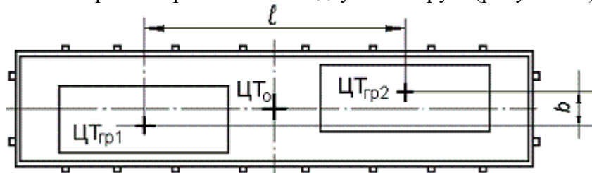
Рисунок 22 - Кососимметричное размещение грузов в вагоне ЦТ ГР1 , ЦТ ГР2 – центры тяжести грузов; ЦТ О – общий центр тяжести вагона с грузом
