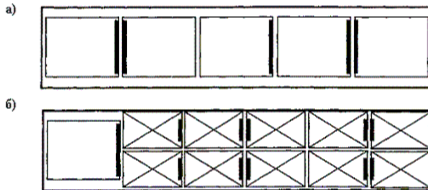
Рисунок 9 – Размещение контейнеров в контейнеровозах с внутренней длиной кузова 13430 мм а – однотипных; б – разнотипных
