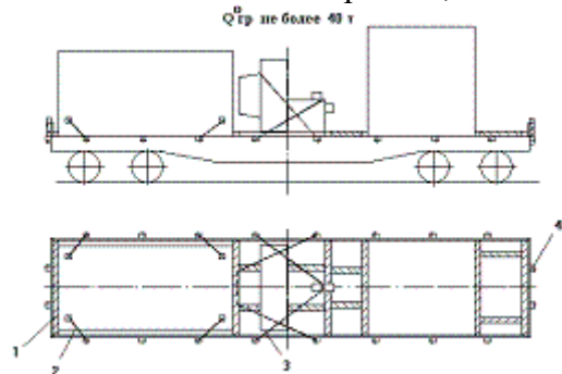
Рисунок 19 1 – брусок упорный; 2 – растяжка; 3 – обвязка; 4 – стойка короткая
