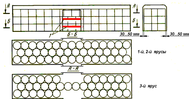
Рисунок 26 – Размещение и крепление рулонов бумаги диаметром 850 мм, шириной 840 мм:
