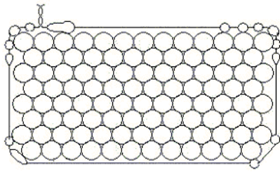
Рисунок 20 – Пакет из круглых лесоматериалов прямоугольной части штабеля
