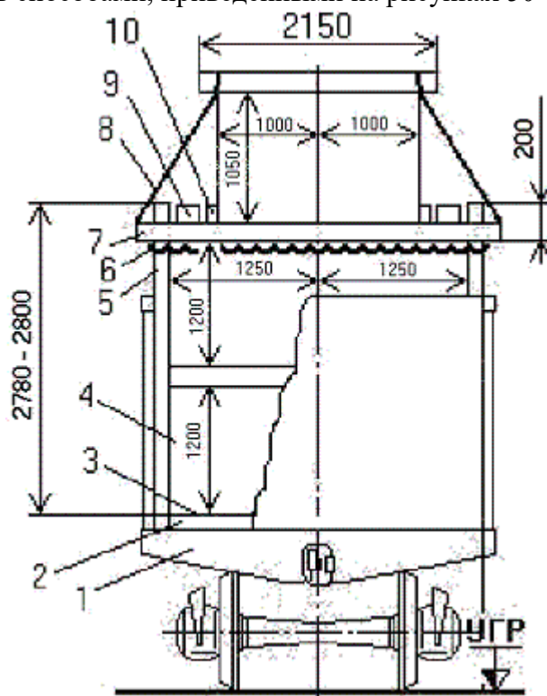
Рисунок 50 – формирование «шапки» по варианту 1 в полувагоне 1 – полувагон; 2 – утолщенная подкладка; 3 – торцовый упор; 4 – пакет прямоугольной части штабеля; 5 – стойка; 6 – скрепление стоек; 7 – удлиненная прокладка; 8 – увязка пакет «шапки»; 9 – распорная доска; 10 – упорный брусок
