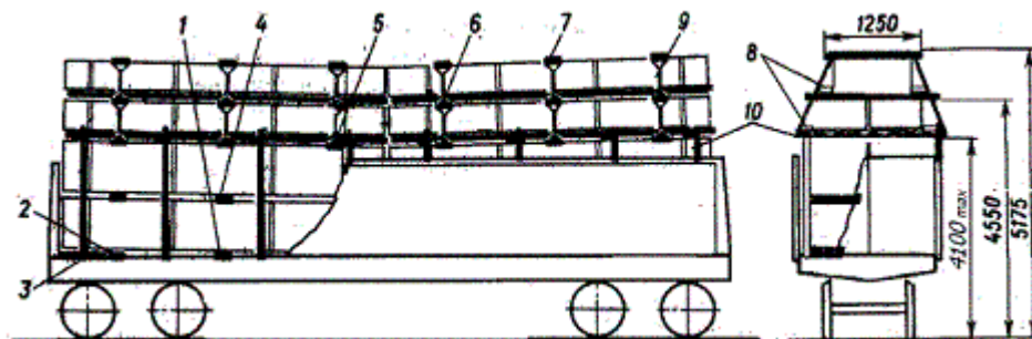
Рисунок 47 – Размещение пакетов пиломатериалов в полувагоне
