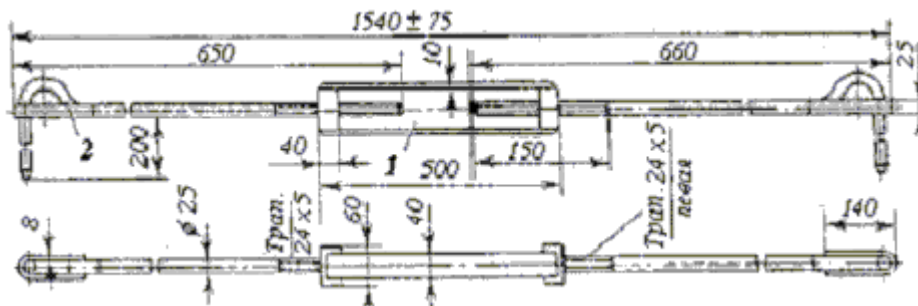
Рисунок 38 – инвентарная стяжка
