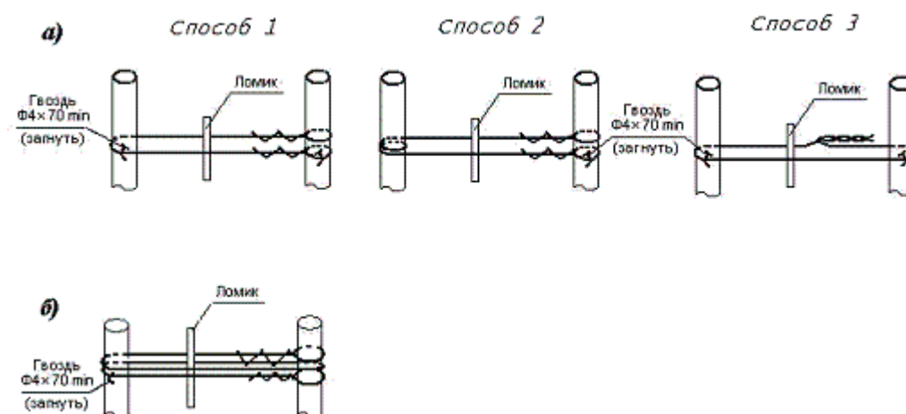
Рисунок 3 – Скрепление стоек
