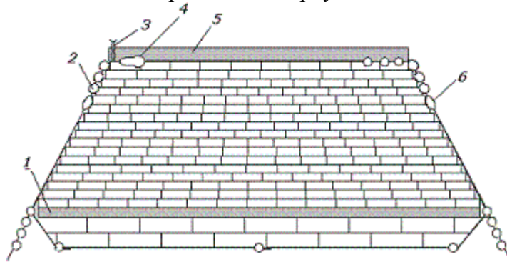
Рисунок 38 – Формирование пакета трапециевидной формы из досок 1 – прокладка; 2 – цепь; 3 – проволочная закрутка; 4 – петлевой замок; 5 – скрепляющая доска; 6 – строповочная проушина
