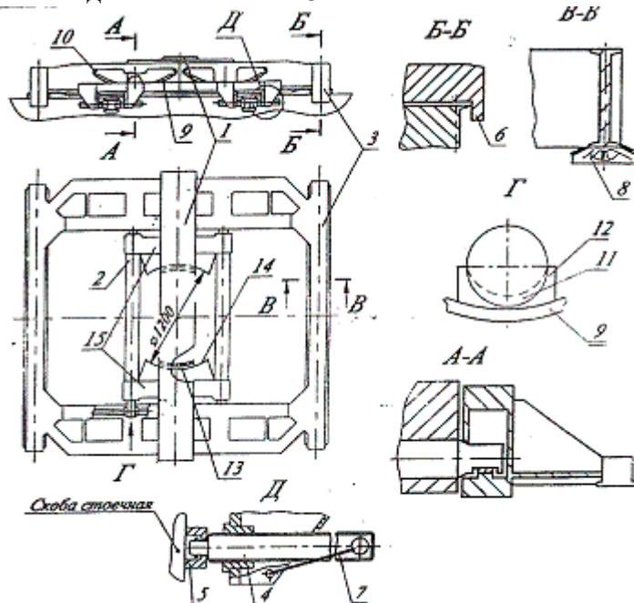
Рисунок 17-Турникетная опора типа Минэнерго
