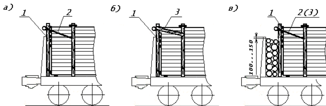
Рисунок 12 – Установка торцовых щитов в полувагоне:
